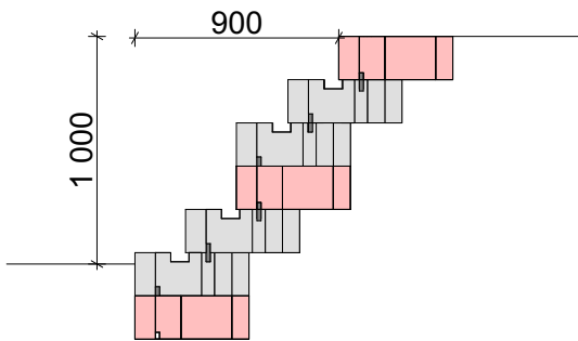
Odklon stěny o 0,90m/1bm výšky
