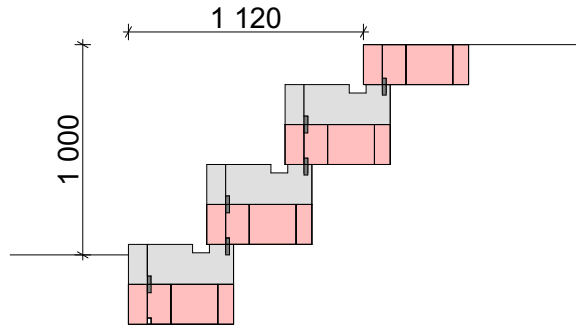
Odklon stěny o 1,12m/1bm výšky
