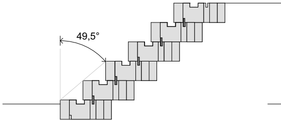
Odklon stěny o 49,5°, tj. 1,11m/1bm výšky
